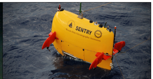
El vehículo autónomo submarino Sentry puede desplazarse a 6,000 metros de profundidad y lleva tanto un sonar multihaz como cámaras de alta definición. Imagen por cortesía de DEEP SEARCH 2017, NOAA-OER/BOEM/USGS.
